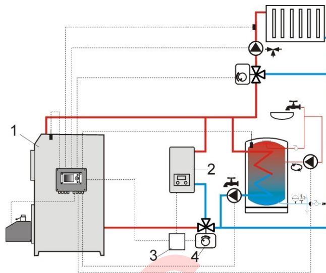
Hüdrauliline skeem täiendava katla avatud-suletud ahelas, milles 1 – juhtseade, 2 – lisakatel, 3 – vahereele, 4 – lülitusklapp (lõpplülititega)
