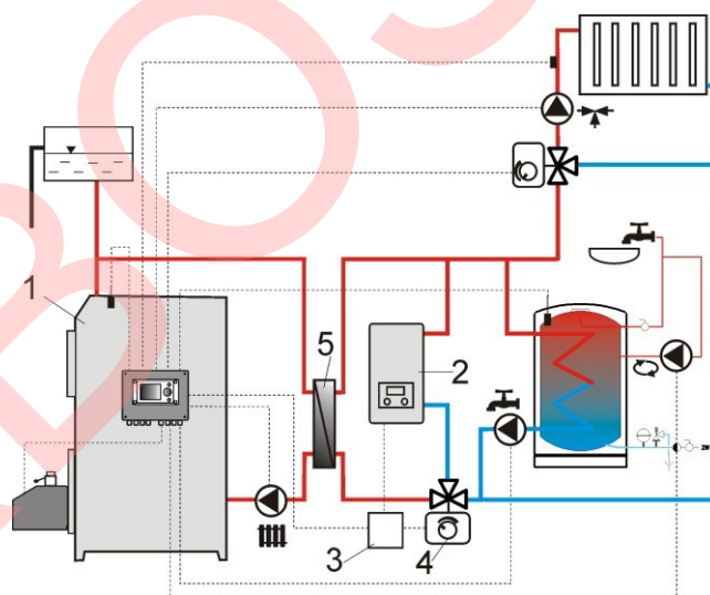
Hüdrauliline skeem täiendava katla avatud-suletud ahelas, milles 1 – juhtseade, 2 – lisakatel, 3 – vahereele, 4 – lülitusklapp (lõpplülititega), 5 – soojusvaheti, soovitatav seade: prioriteet KV = välja lülitatud, soojusvaheti = JAH.
